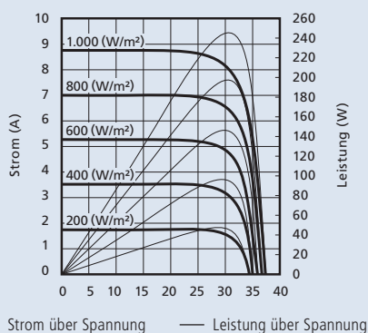
Kennlinien: Strom/Leistung über Spannung (Zelltemperatur: 25 °C)
