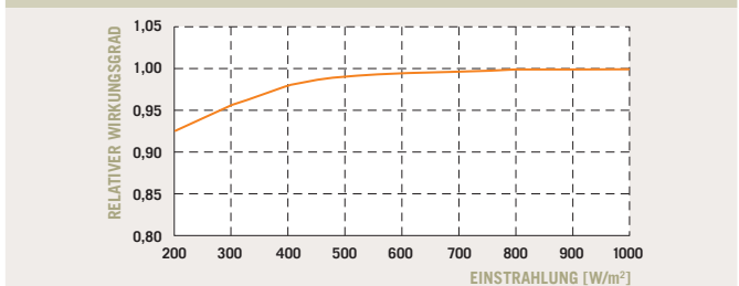
Die typische relative Änderung des Modulwirkungsgrades bei einer Einstrahlung von 200 W/m 2 im Verhältnis zu 1000 W/m 2 beträgt -7 % (gemessen bei 25 °C, AM 1,5 Spektrum).
